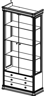
Витрина №321 Цвета: Raiz, Песан, Крема Размеры (ШхВхГ): 970х2145х430
