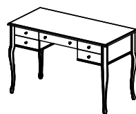
Стол письменный №755 Цвета: Песан, Крема Размеры (ШхВхГ): 1285х800х650
